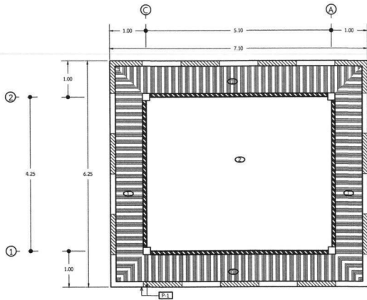
ผังหน้าเพดาน มาตราส่วน 1:75
