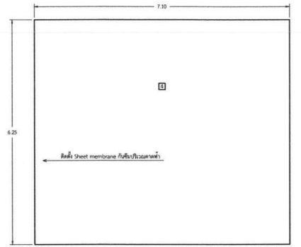
① พื้น ค.ส.บ. ฉนวนกันความร้อน และสีเทา Sheet membrane ผังหลังคา มาตราส่วน 1:75
