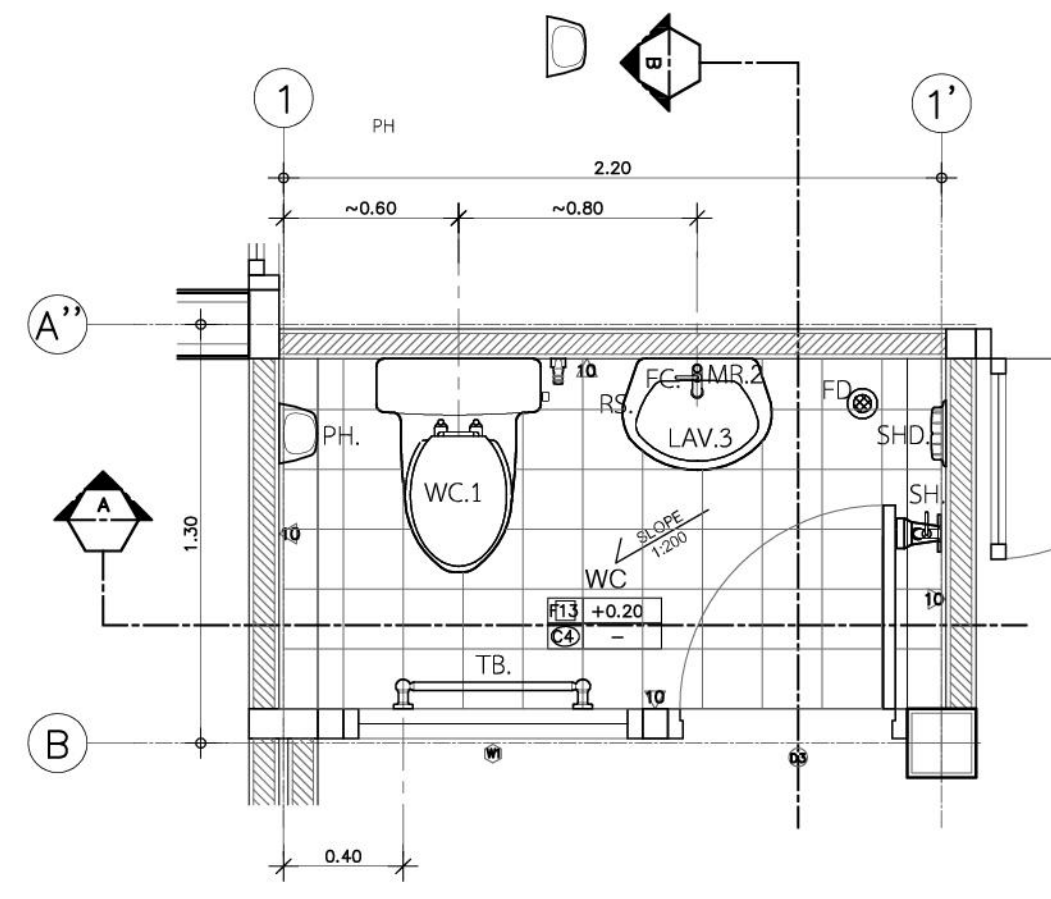
แบบขยายห้องน้ำ มาตราส่วน 1:25
