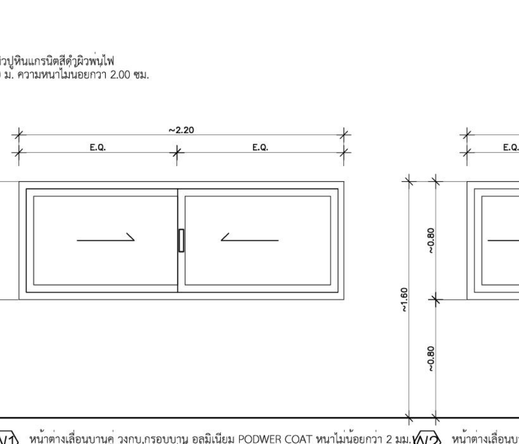
แบบขยายหน้าต่าง มาตราส่วน 1:25
