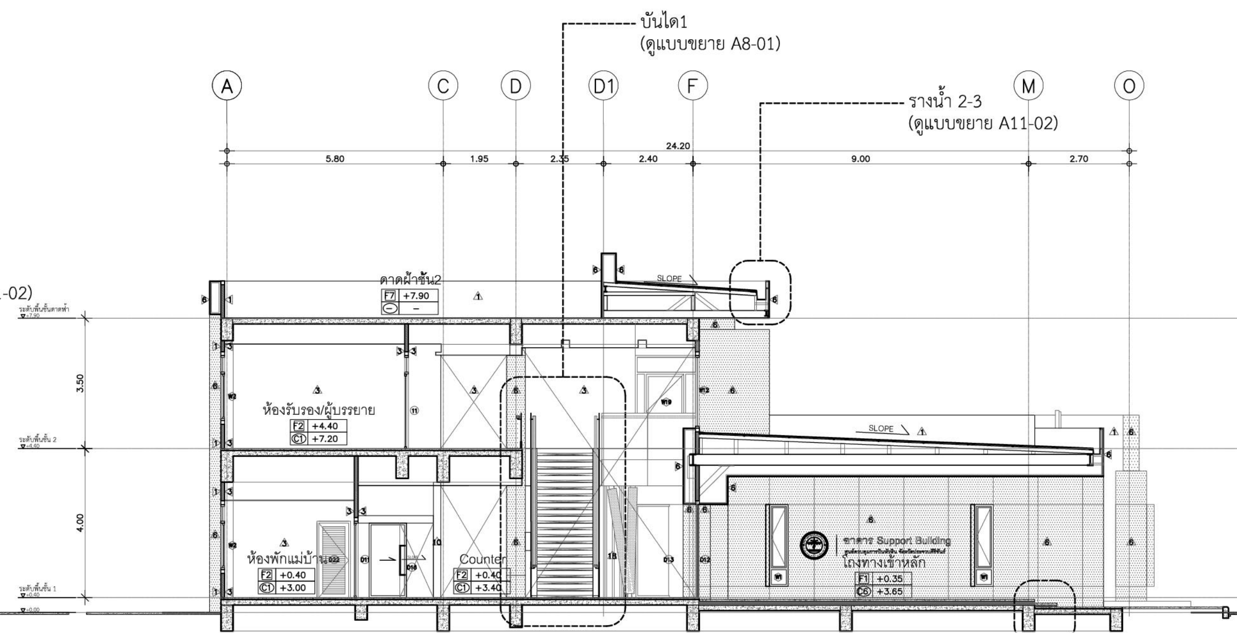
รูปตัด D มาตราส่วน 1:100
