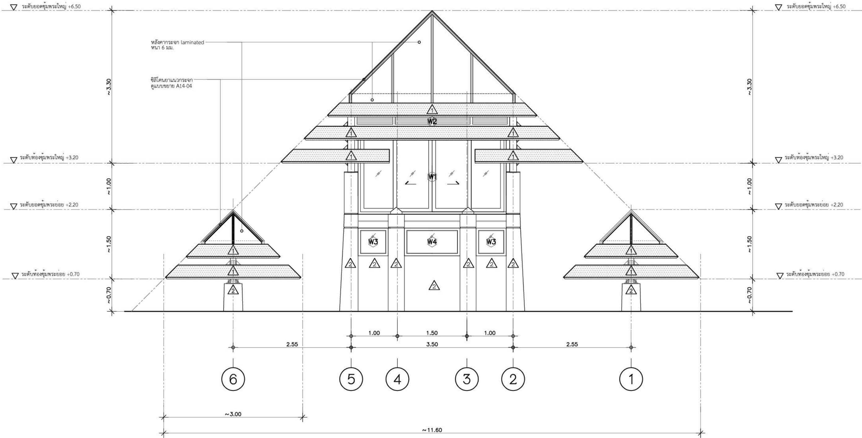
รูปด้าน 3
