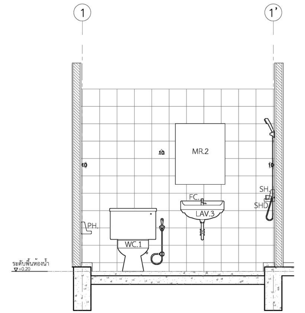
แบบขยายห้องน้ำ มาตราส่วน 1:25
