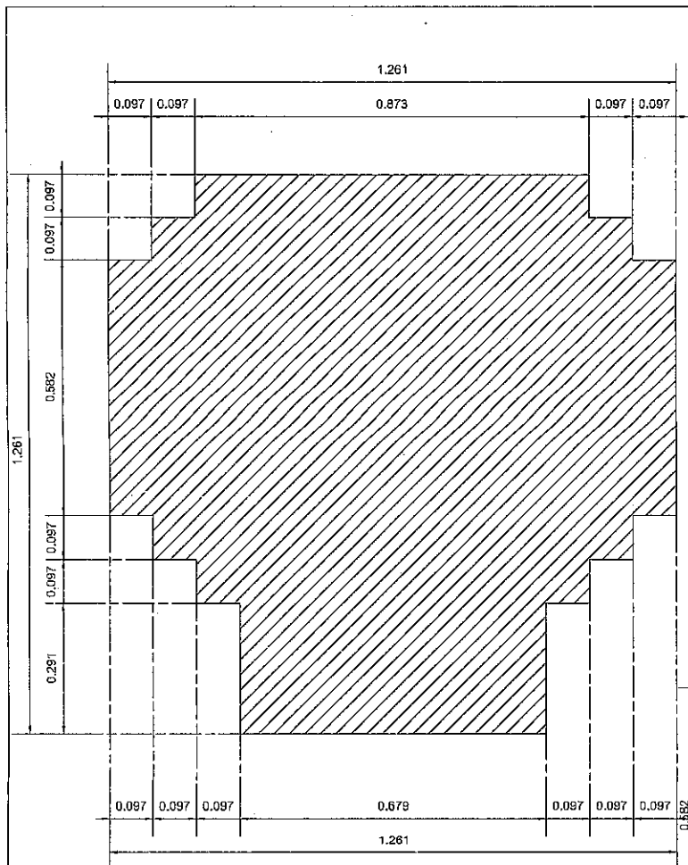
แบบขยายฐานพระ
