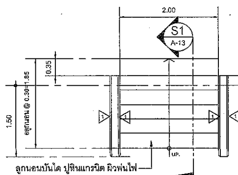
แปลนขยายบันได มาตราส่วน 1:50
