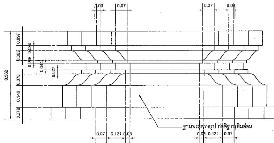
แบบขยายรูปด้านหน้าฐานพระ
