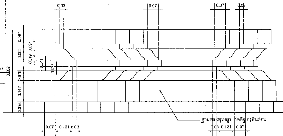
แบบขยายรูปด้านข้างฐานพระ
