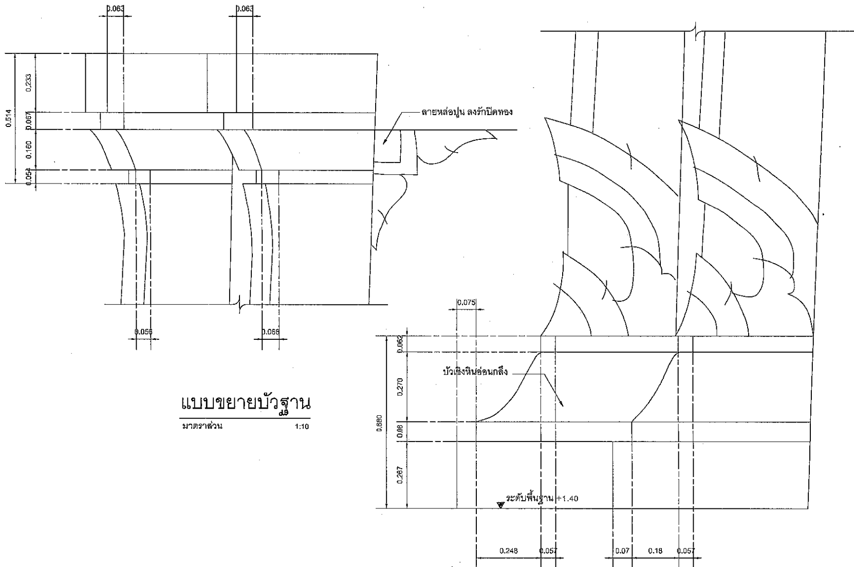
แบบขยายบัวฐาน มาตราส่วน 1:10
