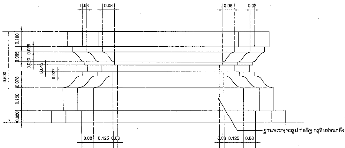
แบบขยายรูปด้านหลังฐานพระ
