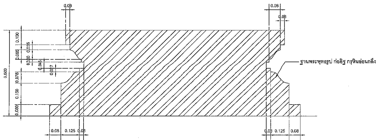
รูปตัดขยายฐานพระ
