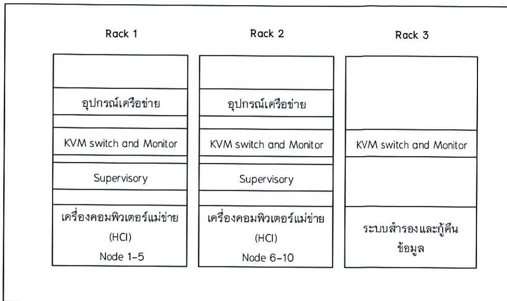
รูปที่ ๓ แสดงการติดตั้งอุปกรณ์ที่จัดหาในโครงการในแต่ละ Rack
