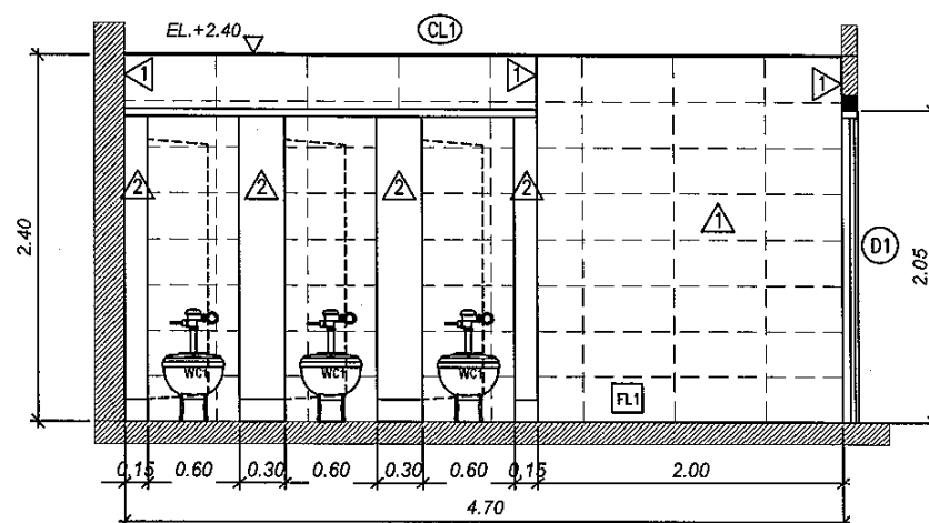
ELEVATION 8
