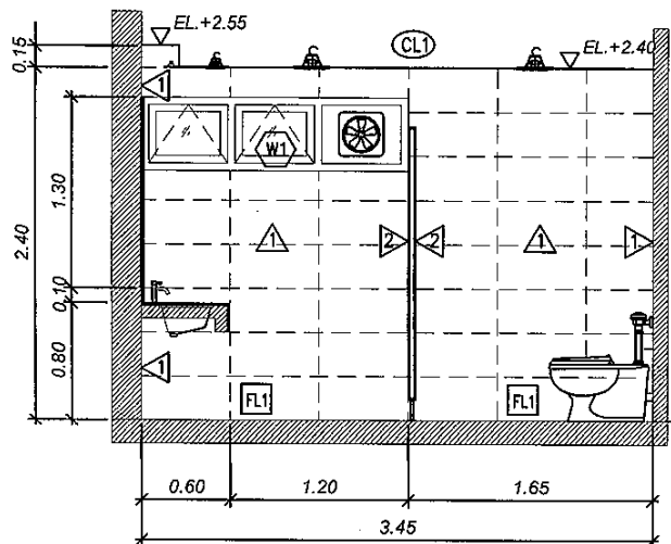
ELEVATION 5
