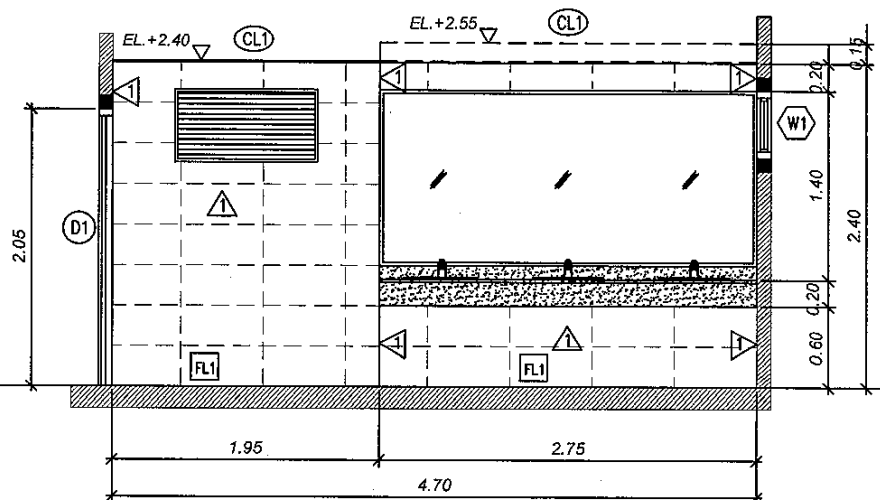
ELEVATION 6
