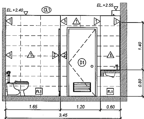
ELEVATION 7
