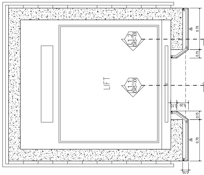
ทางขึ้นลิฟท์ (ช่วงล่างระฆัง) SCALE 1:20
