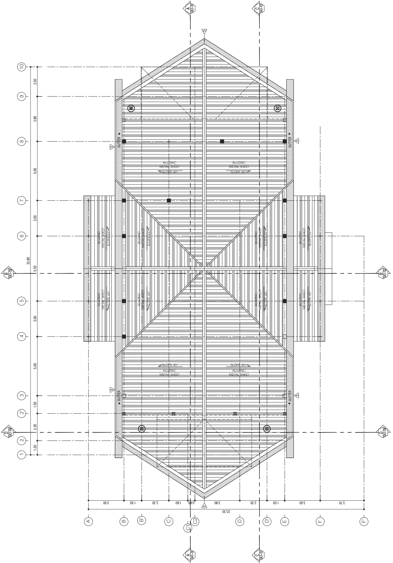
แบบแปลนหลังคา SCALE 1:100
