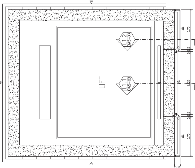
ทางขึ้นลิฟท์ (ช่วงบนระฆัง) SCALE 1:20
