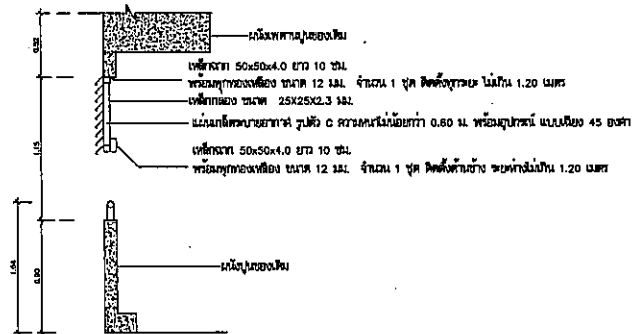
แบบรูปตัดกันสาด SCALE N/A
