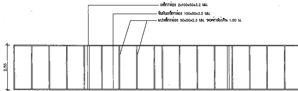
แบบโครงหลังคา 1
