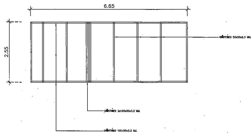
แบบโครงหลังคา 3
