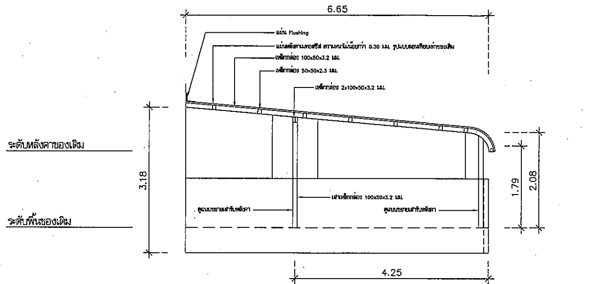
แบบรูปตัดหลังคา 3
