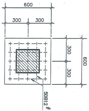
PLAN SCALE 1 : 20
