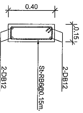
หน้าตัดกลางคาน แบบขยายคาน B1B มาตราส่วน 1:20
