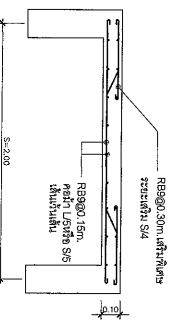
แบบขยาย (SR1) มาตราส่วน 1:20
