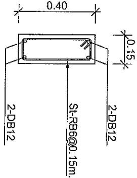
หน้าตัดกลางคาน แบบขยายคาน B1 มาตราส่วน 1:20
