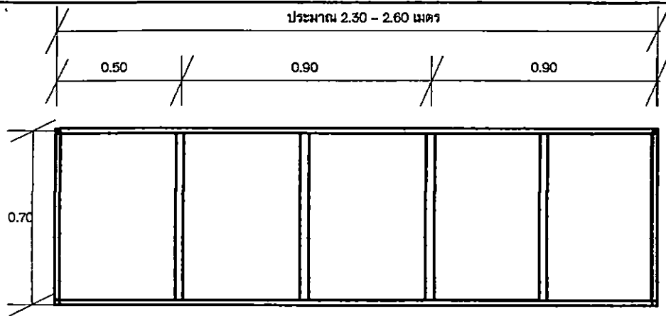
รูปด้านหน้า 1 : 25
