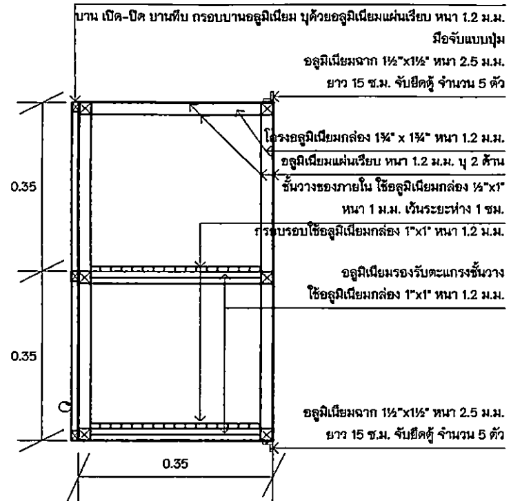
รูปตัดแนว 1-1 / 1:10
