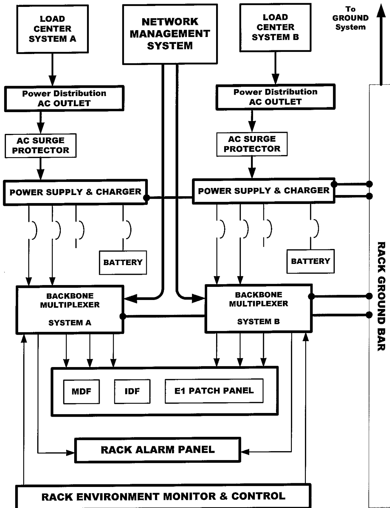
แผนภาพแสดงขอบเขตงานติดตั้งระบบอุปกรณ์ที่ผู้ประสงค์จะเสนอราคาต้องดำเนินการ Diagram 4.1
